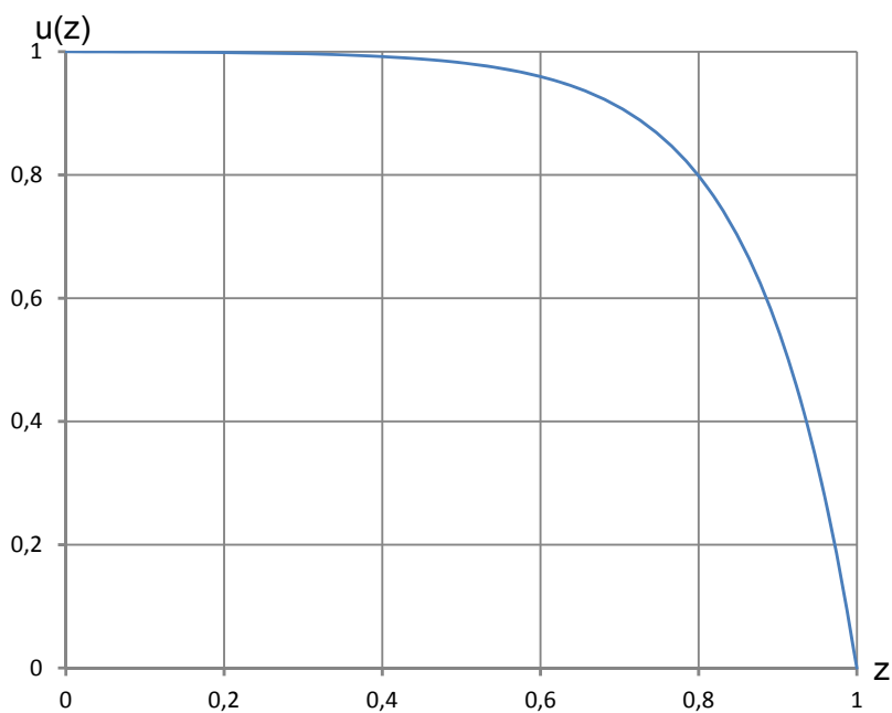
Рис. 4. Стационарное решение
