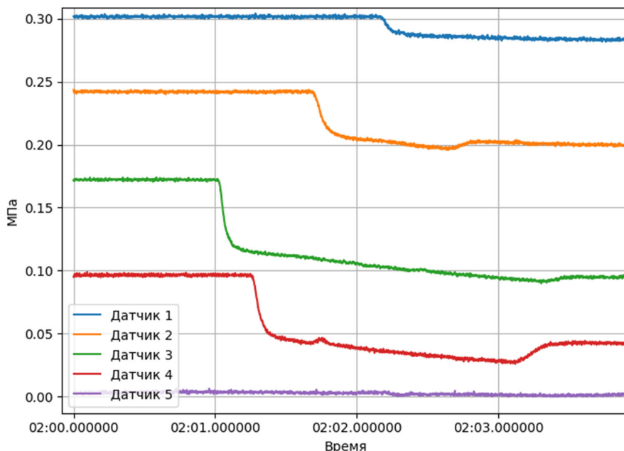
Рис. 3. Результаты измерения давления для возмущения с амплитудой давления в месте возмущений \Delta P^* = 0,12 МПа
