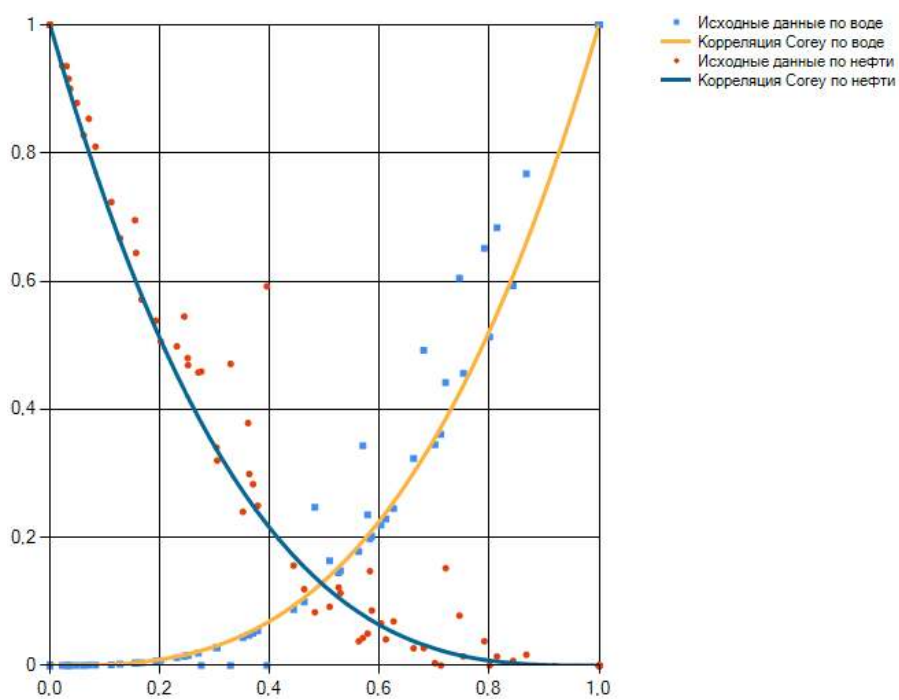
Рис. 2. Модель Кори
