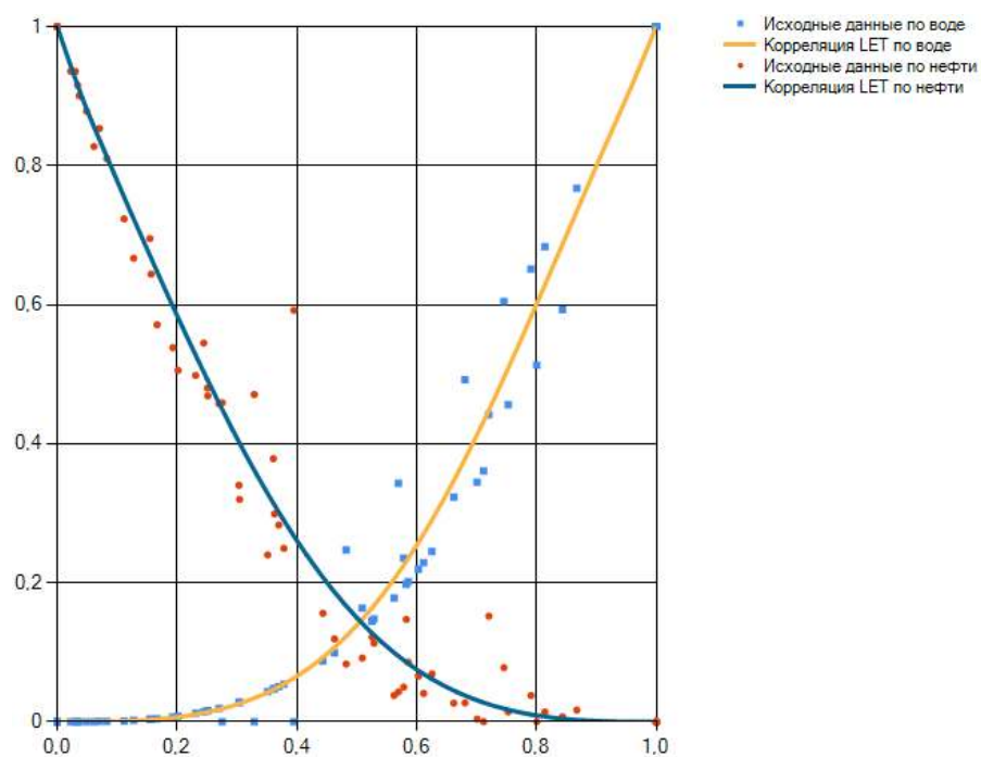
Рис. 1. Модель LET
