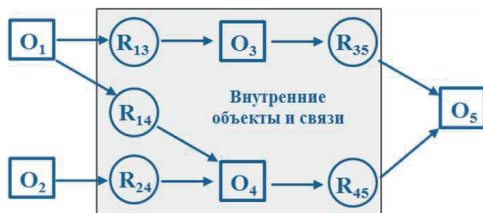
Рис. 3. Представление геолого-математической модели в виде ориентированного двудольного графа
