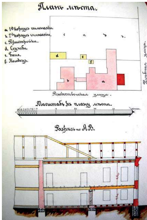
Рис. 11. Проект пристройки к зданию Слободской женской гимназии 1913 г. Ф. 583, оп. 536, ед. хр. 153
