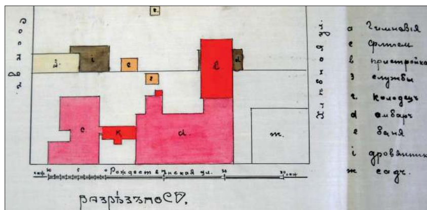
Рис. 4. Проект на пристройку к зданию Словобской женской гимназии. 1909 г. Ф. 583, оп. 532, д. 45
