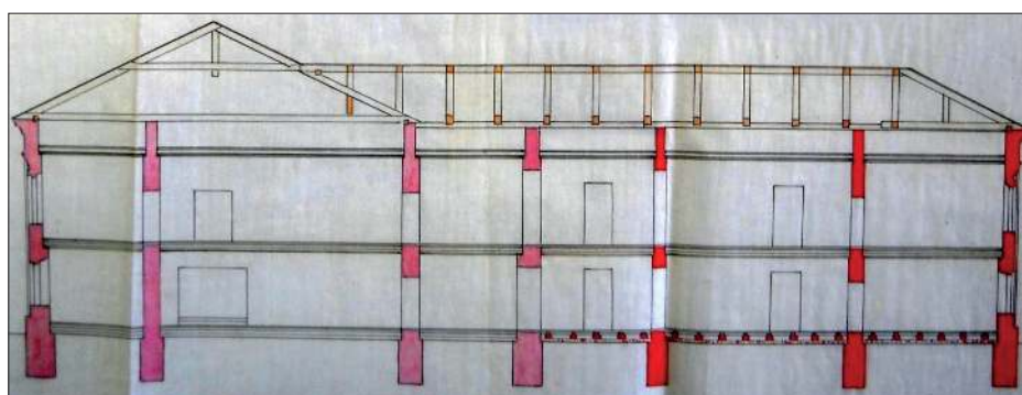
Рис. 6. Проект на пристройку к зданию Словобской женской гимназии. 1909 г. Ф. 583, оп. 532, д. 45
