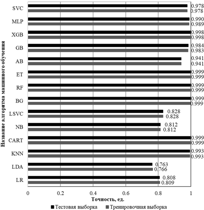
Рис. 9. Оценка точности различных алгоритмов машинного обучения
