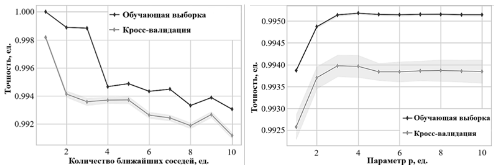
Рис. 15. Оптимизация гиперпараметров алгоритма «К-ближайших соседей»
