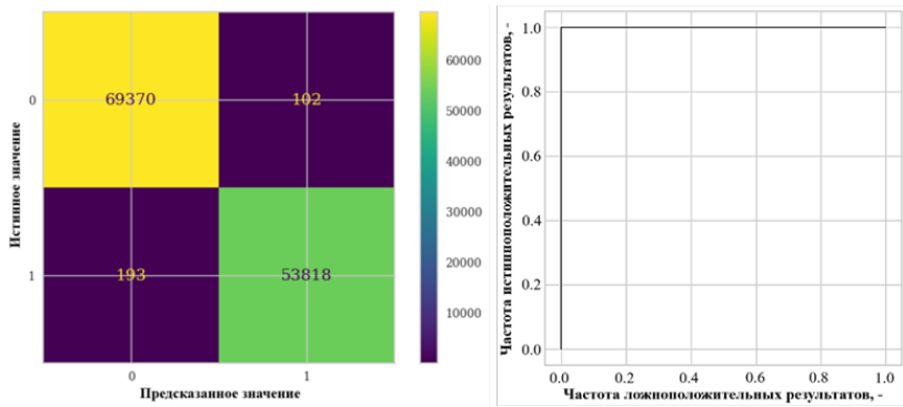
Рис. 17. Матрица неточностей (слева) и кривая ROC (справа) для алгоритма «K-ближайших соседей» для тестовой выборки
