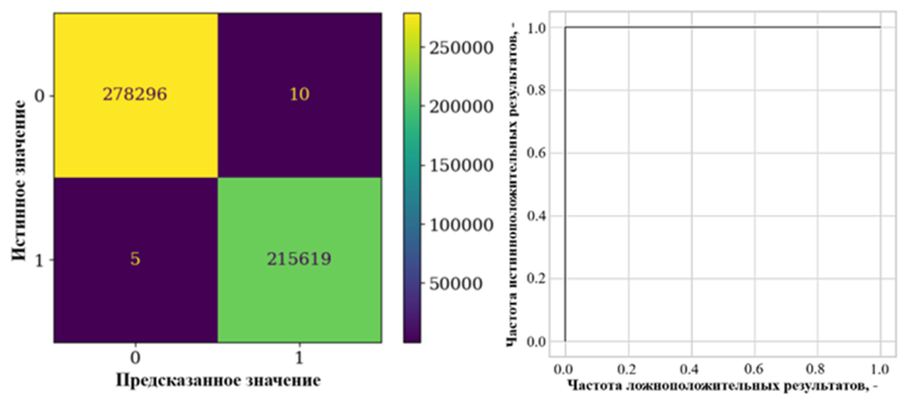
Рис. 12. Матрица неточностей (слева) и кривая ROC (справа) для алгоритма «дерево принятия решений» для обучающей выборки Fig. 12. Inaccuracy matrix (left) and ROC curve (right) for the “decision tree” algorithm (training data sample)
