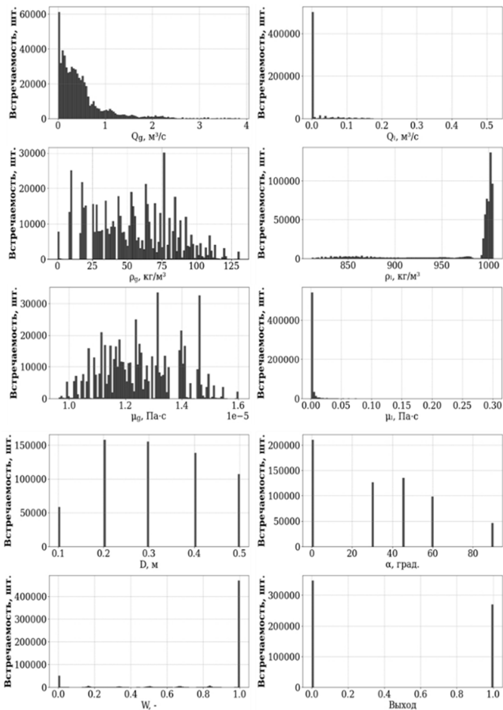
Рис. 2. Частота встречаемости определяющих параметров выборки Fig. 2. Frequency occurrence of determining parameters (factors) of the data sample
