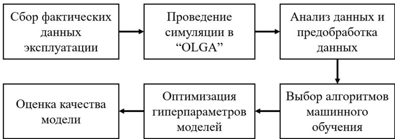
Рис. 1. Блок-схема методологии, представленной в данной работе
