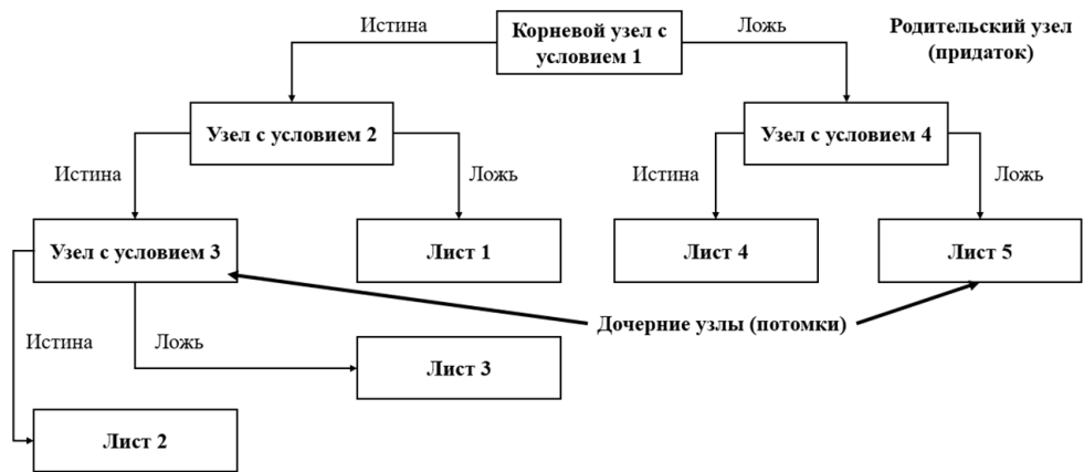
Рис. 10. Принципиальная схема работы алгоритма «дерево принятия решений» Fig. 10. Principal scheme of the „decision tree“ algorithm
