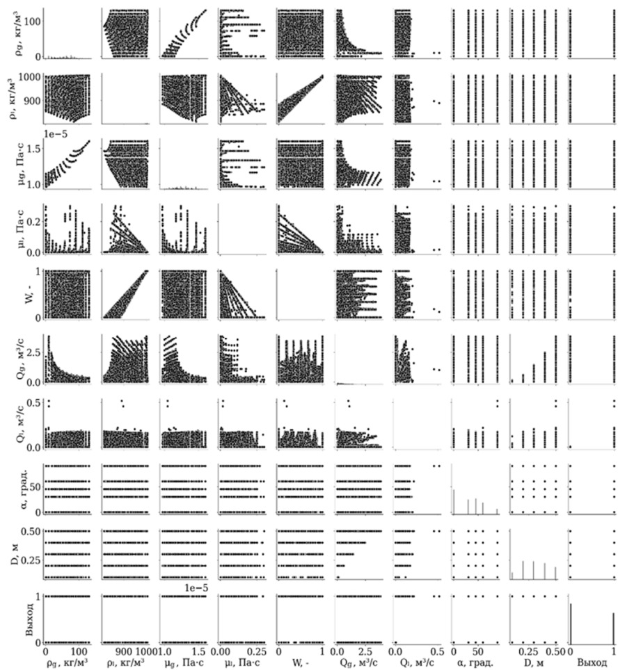
Рис. 6. Диаграмма рассеивания для определяющих параметров (факторов) выборки
