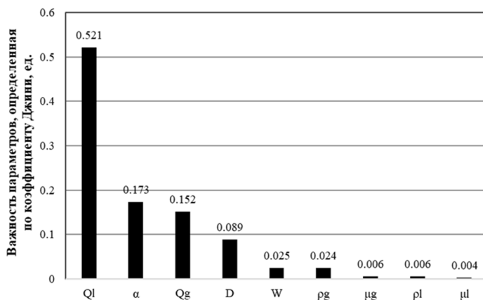
Рис. 14. Важность параметров, основанная на коэффициенте Джини
