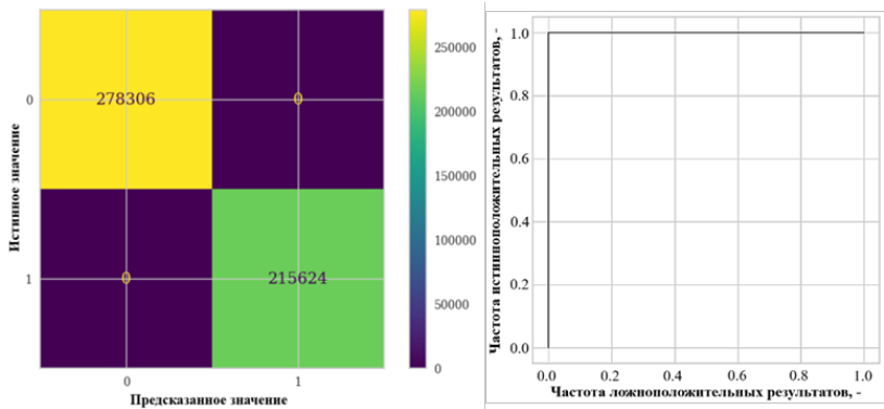
Рис. 16. Матрица неточностей (слева) и кривая ROC (справа) для алгоритма «К-ближайших соседей» для обучающей выборки
