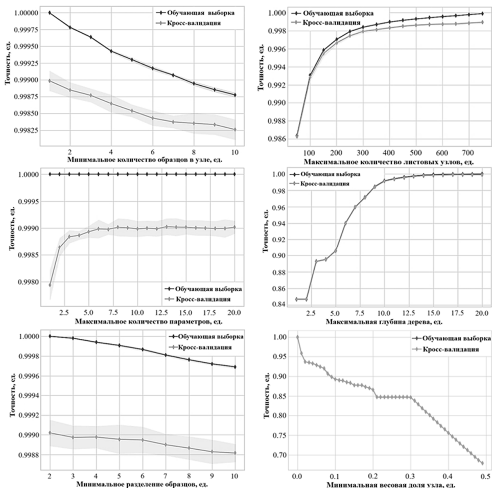
Рис. 11. Оптимизация гиперпараметров алгоритма «дерево принятия решений»
