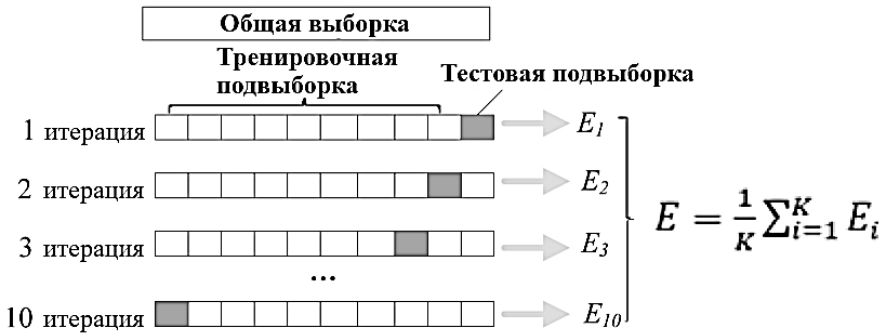
Рис. 8. Принцип работы метода кросс-валидации
