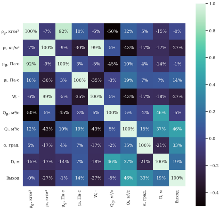
Рис. 5. Корреляционная матрица в определяющих параметрах выборки Fig. 5. Correlation matrix in determining parameters (factors) of the data sample
