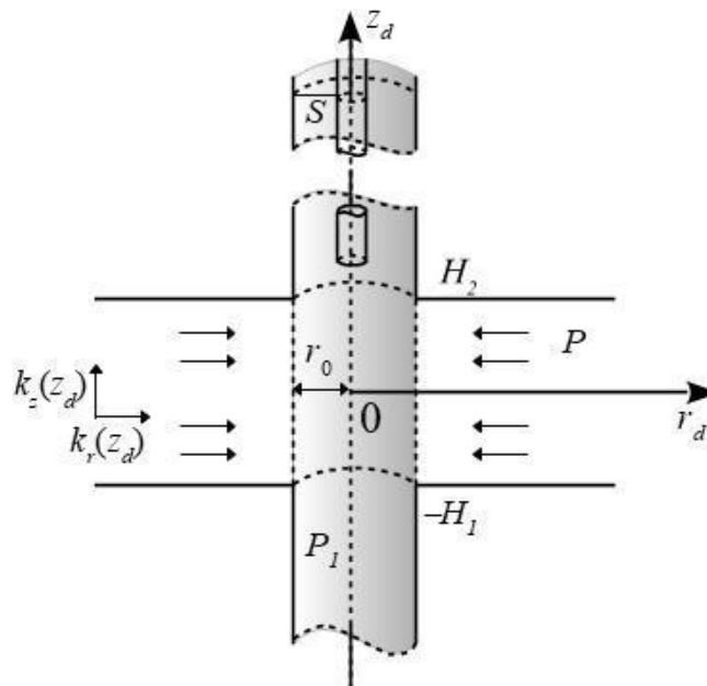
Рис. 1. Геометрия задачи
