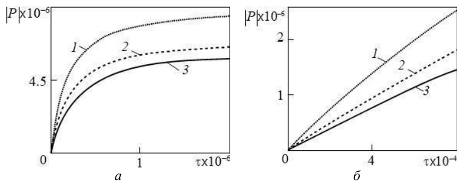
Рис. 3. Зависимость давления от безразмерного времени на различных расстояниях от скважины: 1 — r = 1 , 2 — 5, 3 — 10
