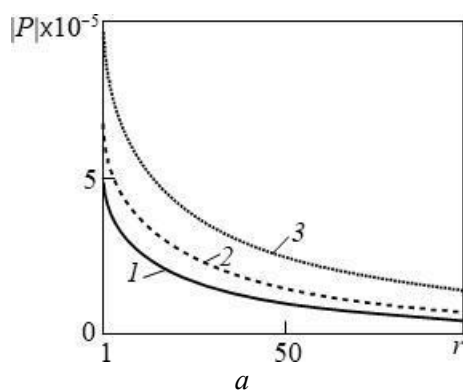
Рис. 4. Зависимость давления от радиальной координаты для различных времен.
