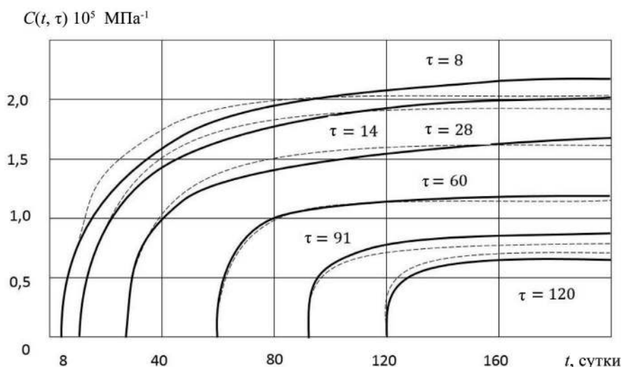
Рис. 1. Экспериментальные и теоретические кривые мер ползучести бетонных образцов разного возраста \tau : — — — экспериментальные данные; - - - - - аппроксимация эксперимента выражением (8)
